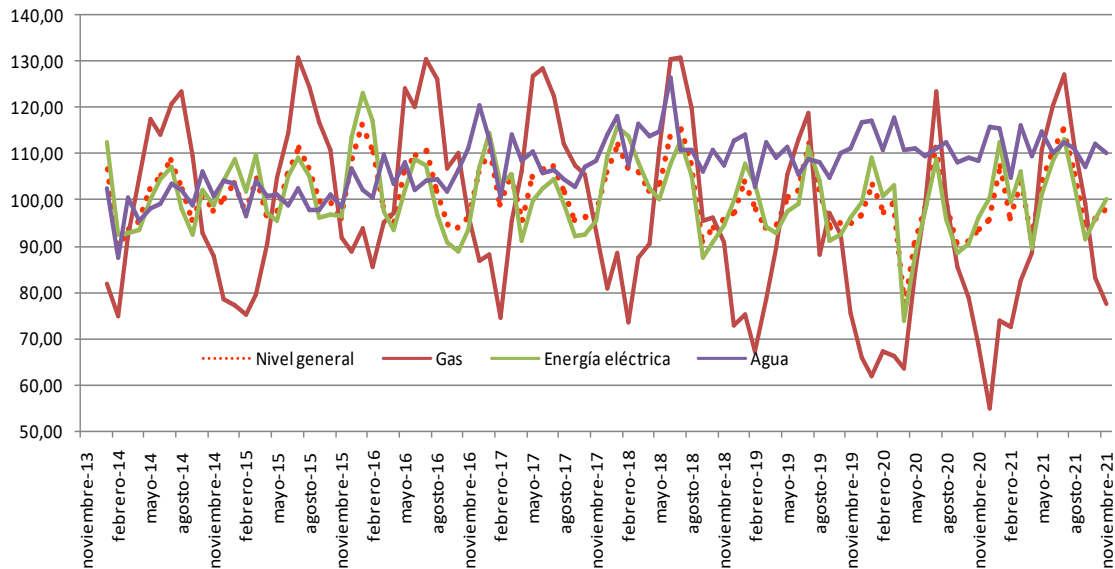
Gráfico 2. Índice de Servicios Públicos. Nivel general y tipos de servicios. Serie original Base 2014=100. Período: enero 2014 – noviembre 2021.
